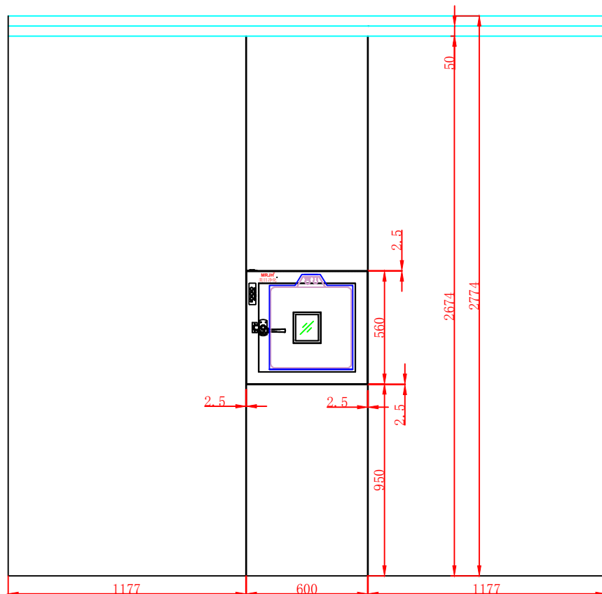
正视图
