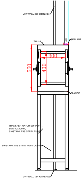
侧视（剖面）图
