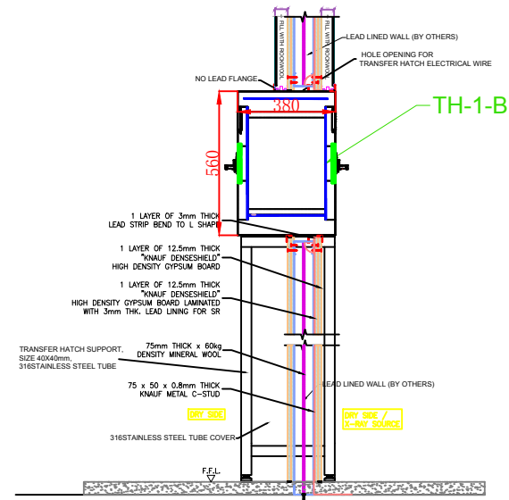
侧视（剖面）图
