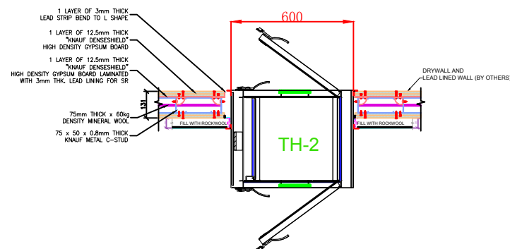
俯视（剖面）图
