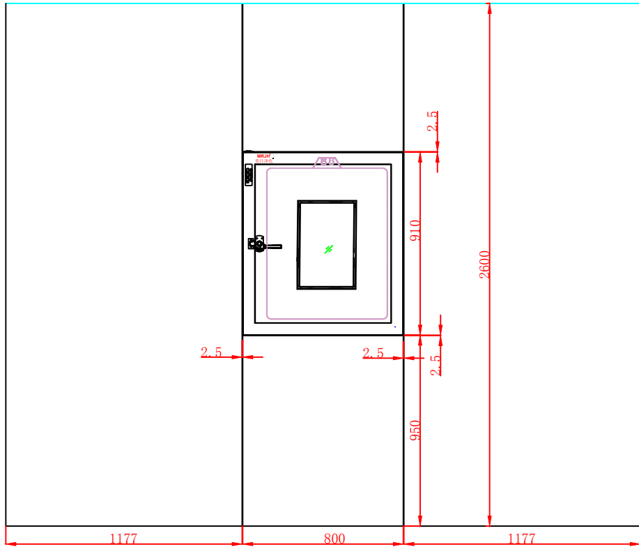
正视图
