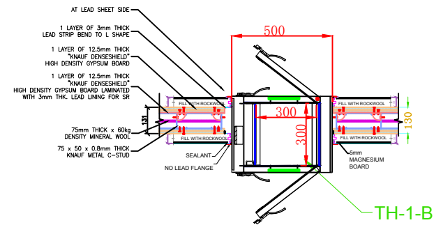
俯视（剖面）图
