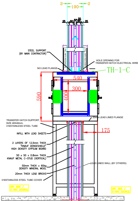
侧视 <剖面> 图
