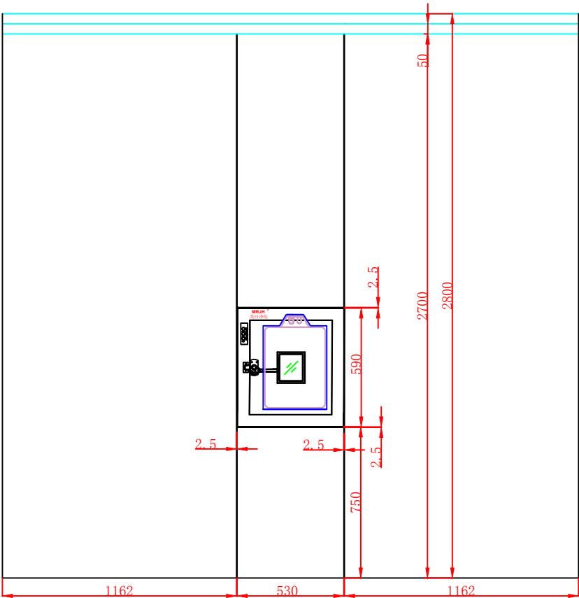
正视图
