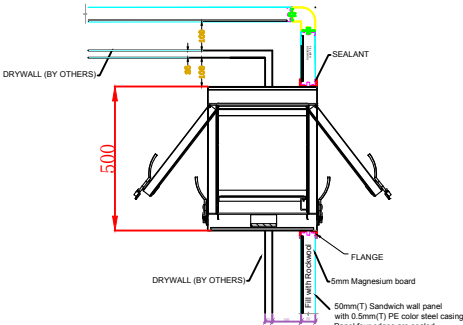
俯视（剖面）图
