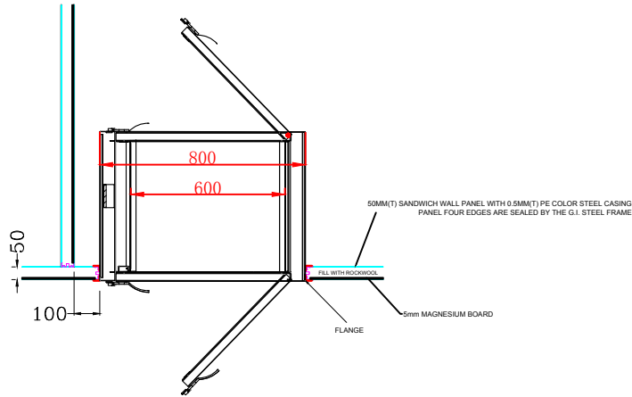
俯视（剖面）图
