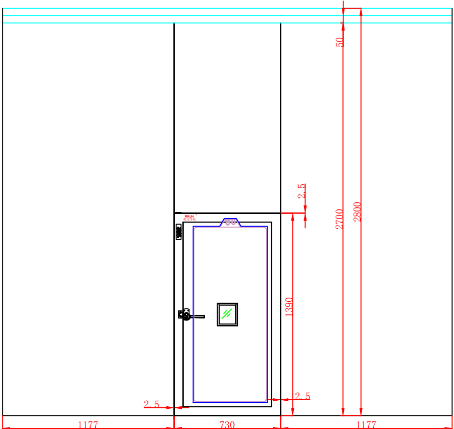
正视图
