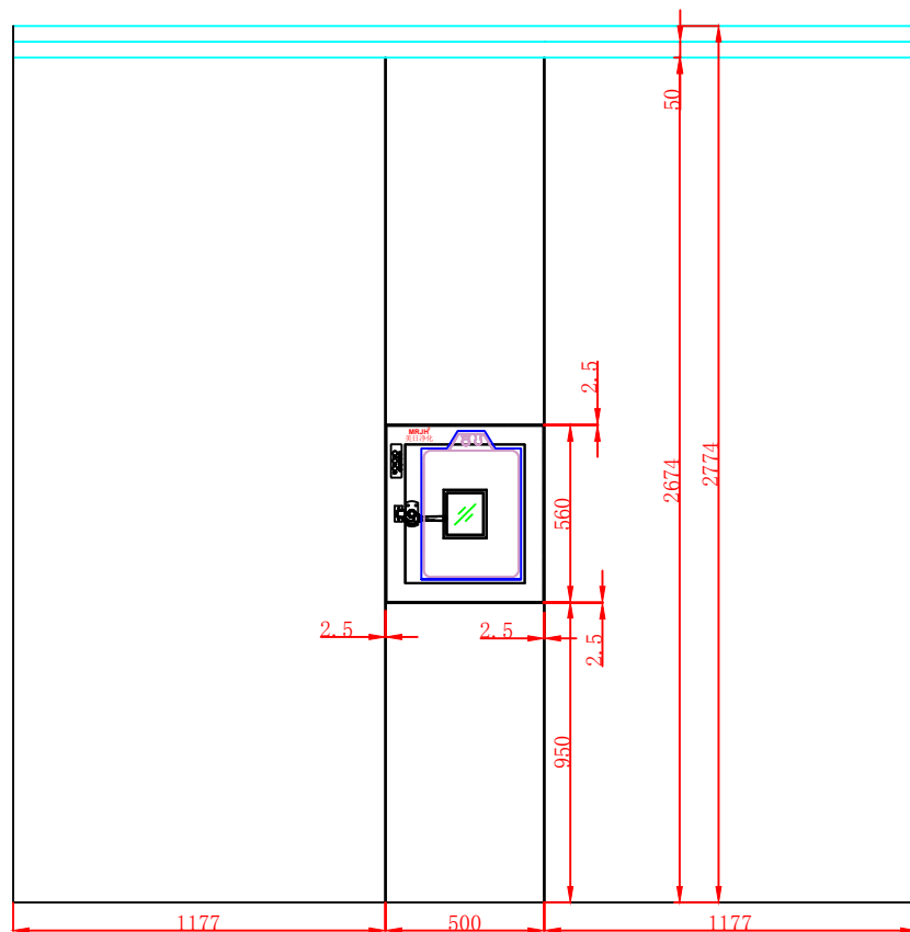
正视图
