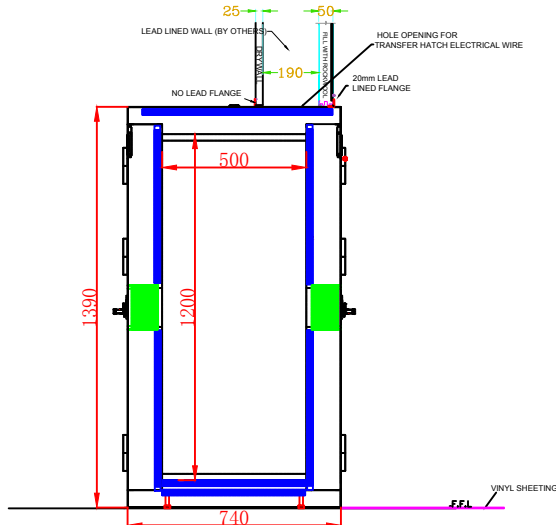
侧视〈剖面〉图
