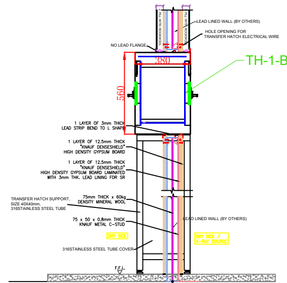
侧视（剖面）图
