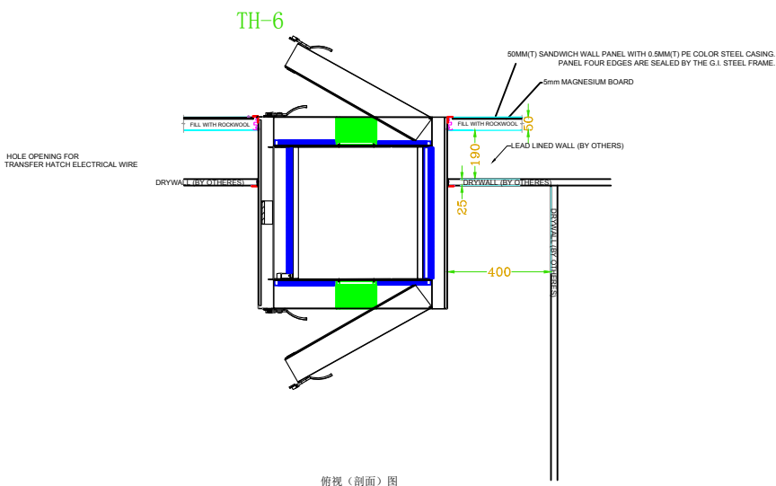
俯视〈剖面〉图
