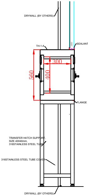
侧视（剖面）图
