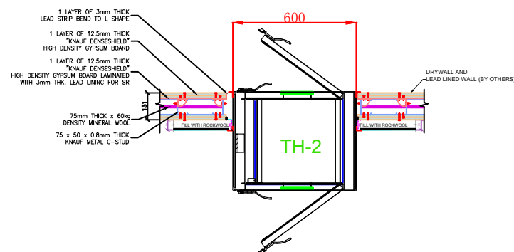
俯视〈剖面〉图
